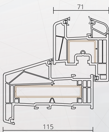
Verdiept systeem met aanslag
