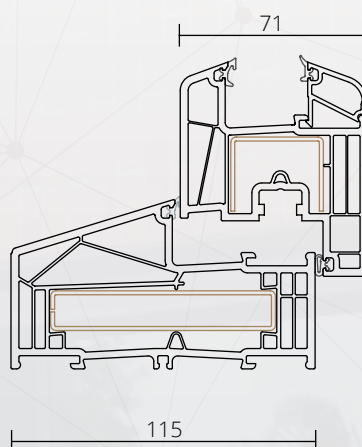
Verdiept systeem zonder aanslag
