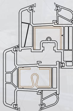
T-kozijnprofiel
