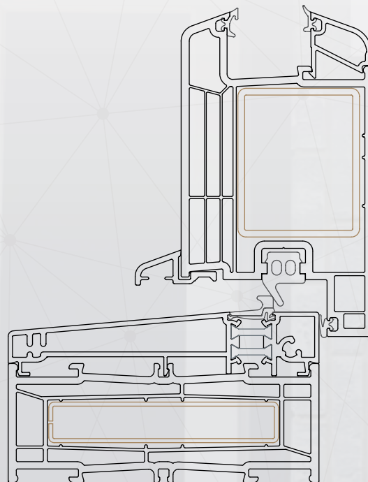
Deur NL71 Arcade naar binnen draaiend
