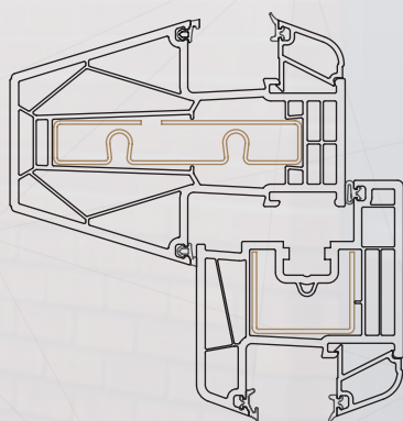
Stijl-, kalfverbinding
