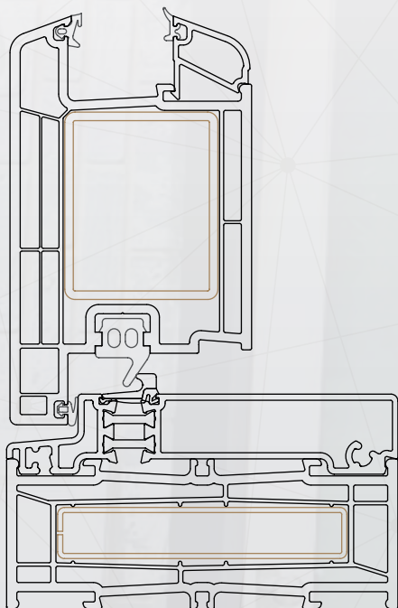
Deur NL71 Arcade naar buiten draaiend
